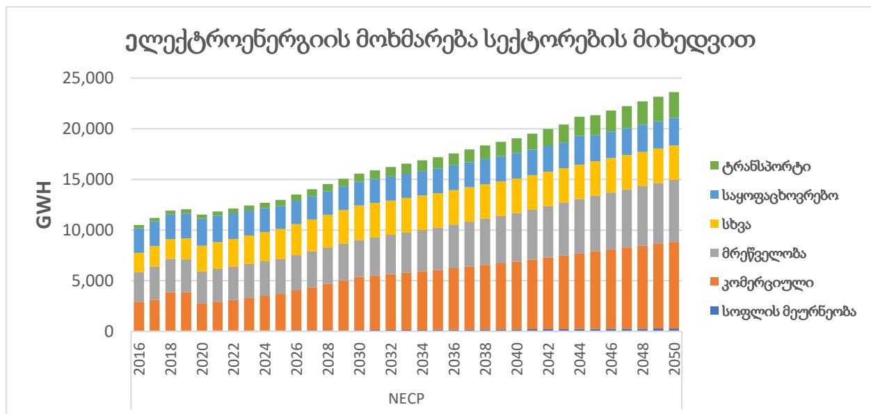
გრაფიკი 5. ელექტროენერგიის მოხმარების პროექცია NECP სცენარში
