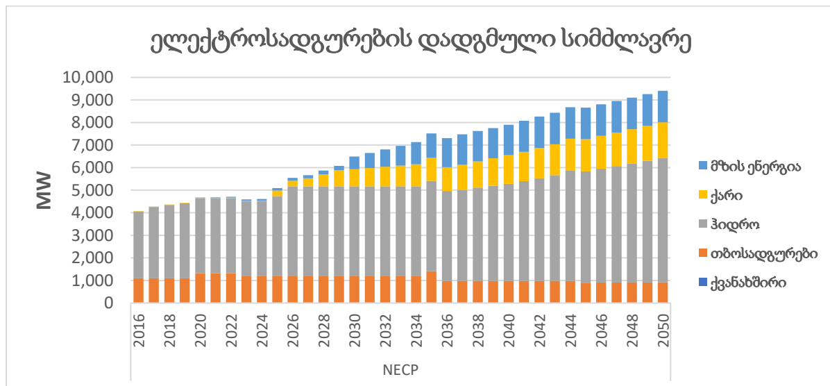
გრაფიკი 6. ელექტროენერგიის გენერაციის სადგურების სიმძლავრის ცვლილება დაგეგმვის პერიოდის განმავლობაში
